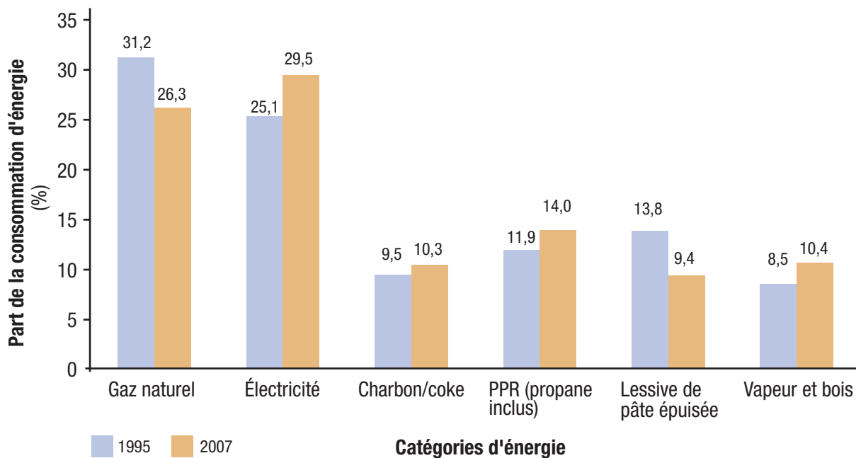
Figure 4. Part de la consommation d'énergie dans le secteur manufacturier, selon la catégorie d'énergie, 1995 et 2007
