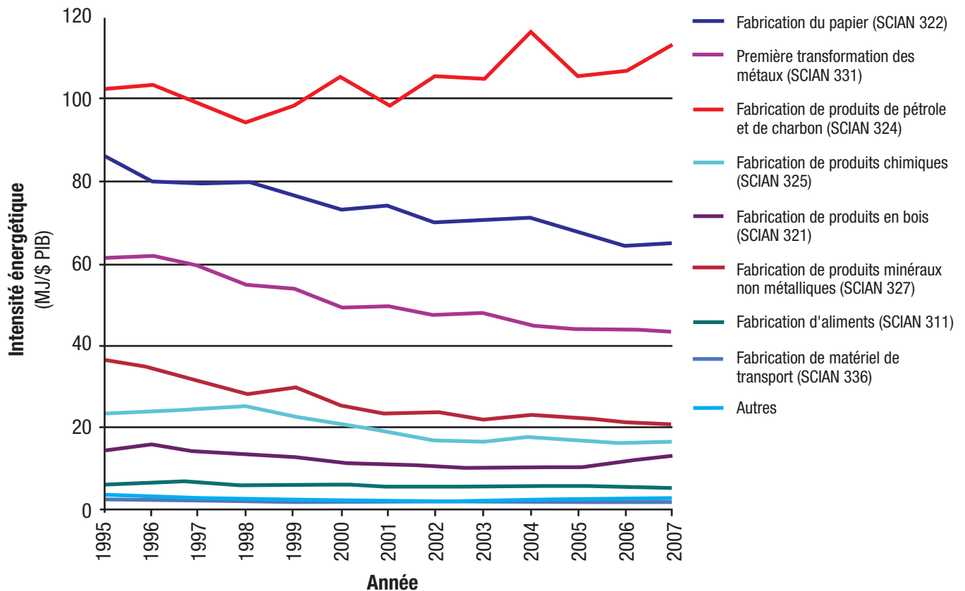
Figure 2. Intensité énergétique dans les sous-secteurs sélectionnés, de 1995 à 2007
