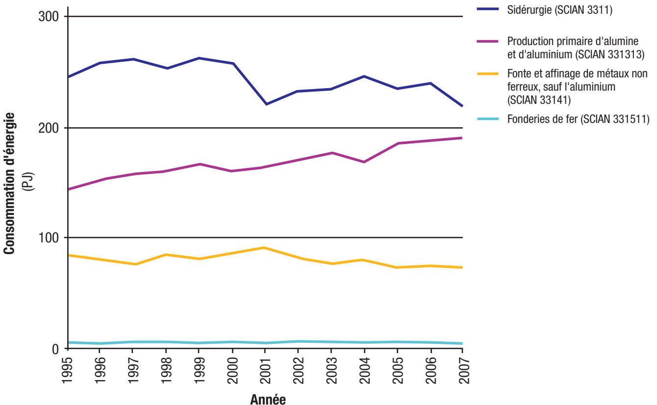
Figure 11. Consommation d'énergie dans les industries de première transformation des métaux sélectionnées, de 1995 à 2007
